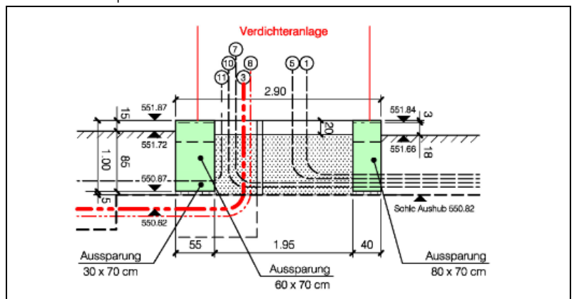
Fundamente Verdichteranlage
