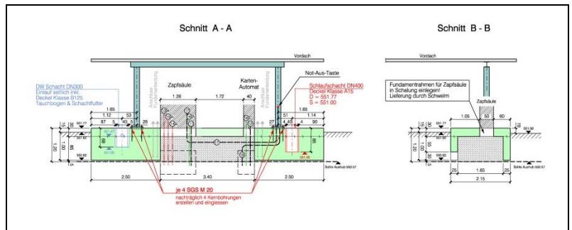
Fundament Zapfsäule und Kartenautomat
