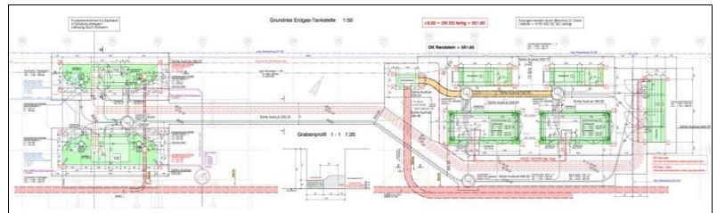
Grundriss Erdgas-Tankstelle
